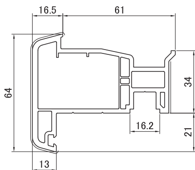
8080 Штульп 64 мм
