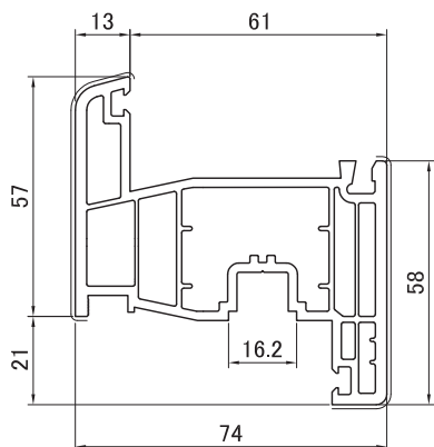
8095 Створка оконная 78 мм
