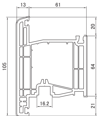
8079 Створка дверная 105 мм
