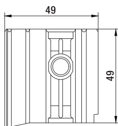
8496 Соединитель импоста
