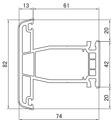
8037 Импост 82 мм
